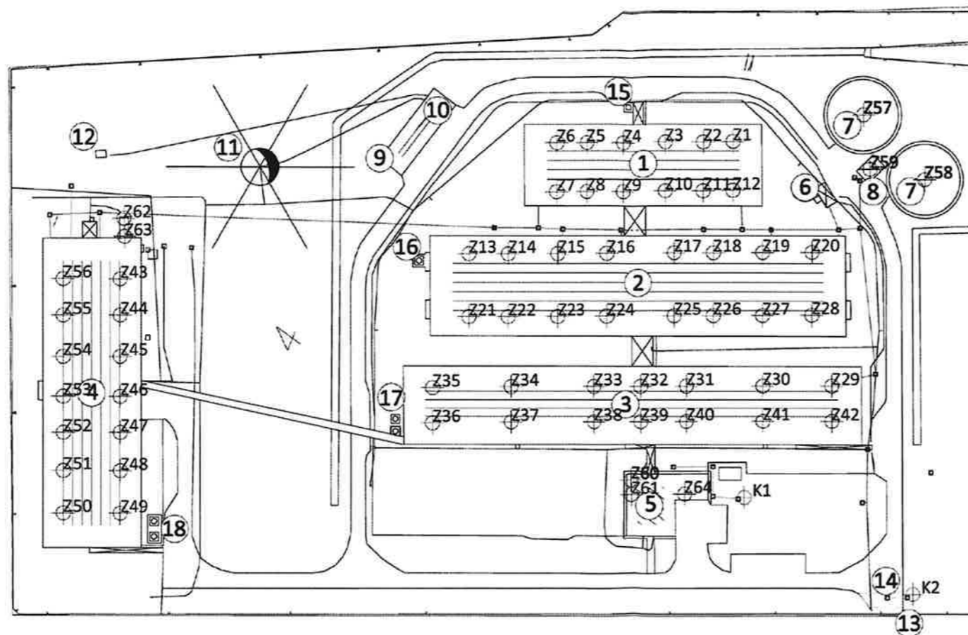
Prilog 1. Situacija sa prikazom objekata, mjesta emisija i sustava vodoopskrbe i odvodnje na lokaciji farme Malo Kneževo.
